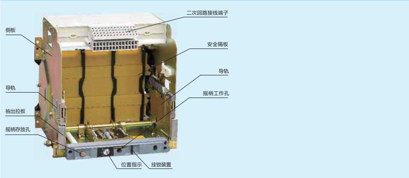
NA8G-3200 抽屉座结构
