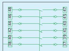
IV、三开三闭触头
