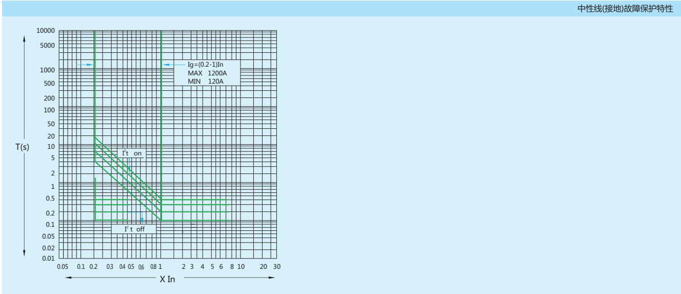
中性线(接地)故障保护特性
