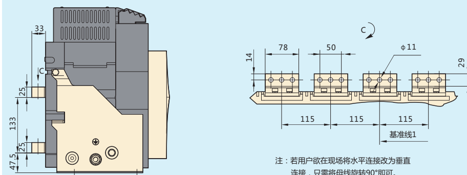
NA8G-4000(In=1000A~2500A)固定式断路器安装尺寸(用户自行完成垂直接线)
