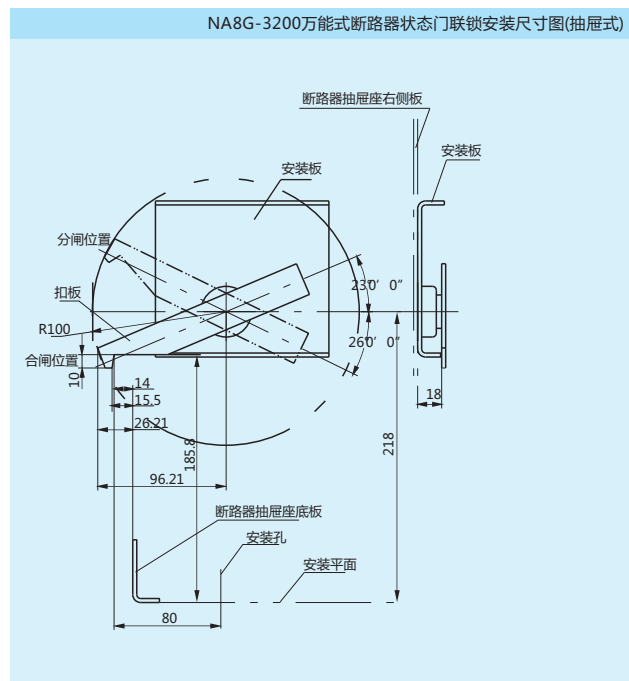
NA8G-3200万能式断路器状态门联锁安装尺寸图(抽屉式)
