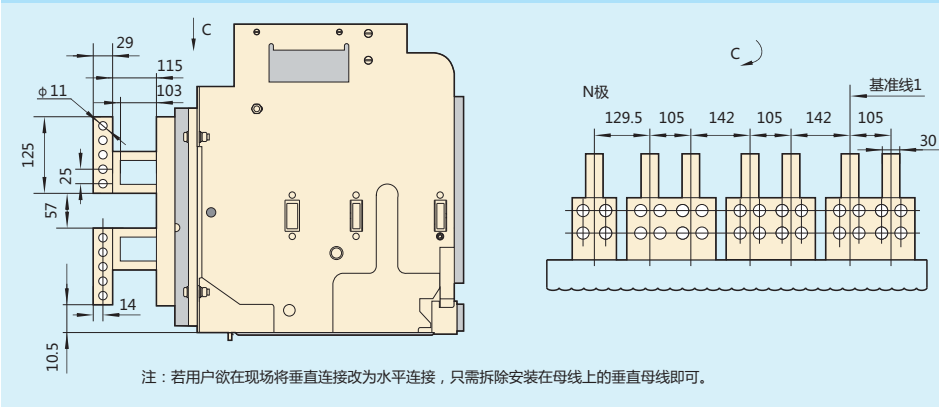
NA8G-6300(In=4000A~5000A)抽屉式断路器安装尺寸(用户自行完成垂直连接)
