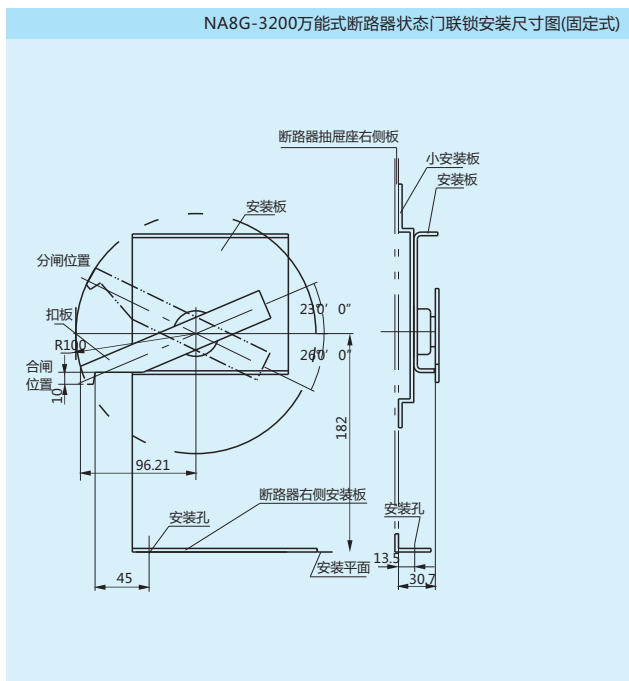
NA8G-3200万能式断路器状态门联锁安装尺寸图(固定式)
