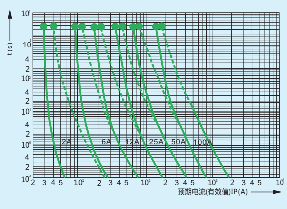
RT28圆筒形帽熔断器特性曲线
